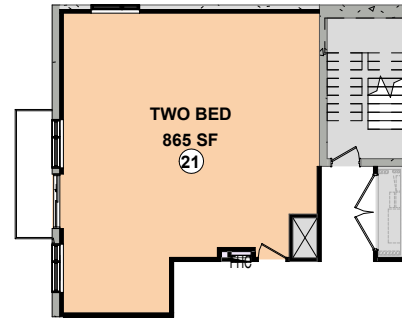
4P COR STA MODULE - OPT 2 KEY PLAN
