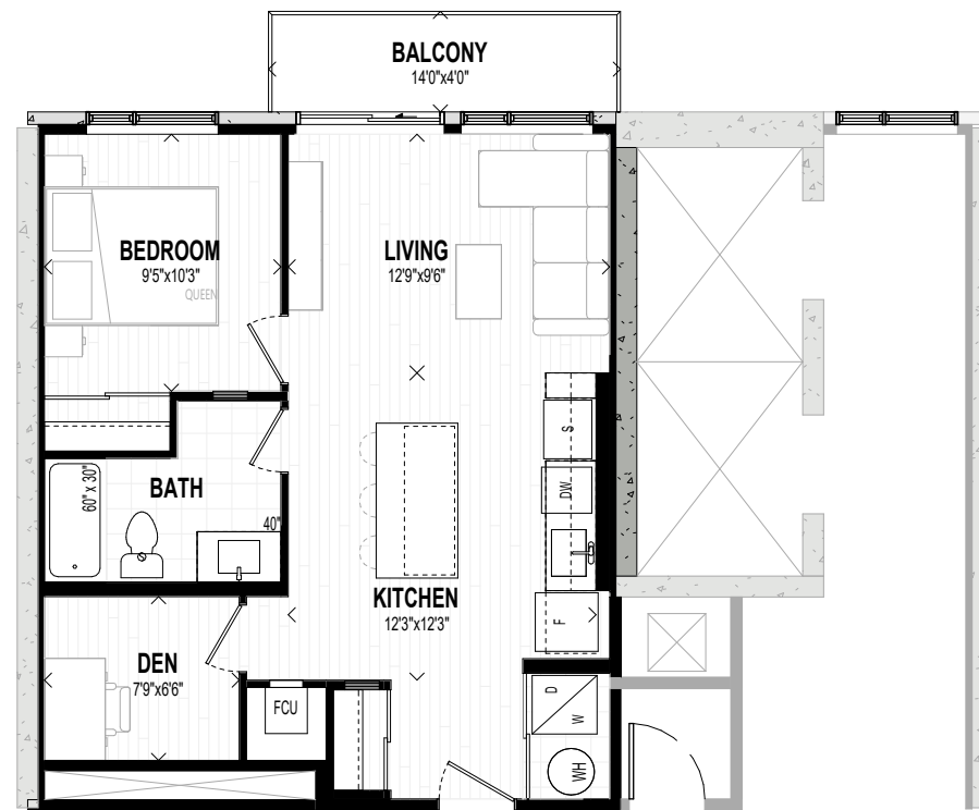
23 ONE BEDROOM + DEN 1 : 100
