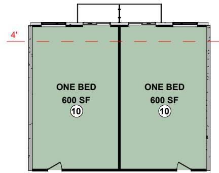
4P DEEP MODULE - OPT 1 KEY PLAN
