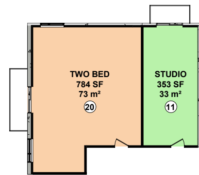
4P COR MODULE - OPT 4
